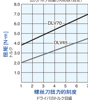
输出扭矩刻度对照表(目标) 出力トルク目盛り対応表(目安)
